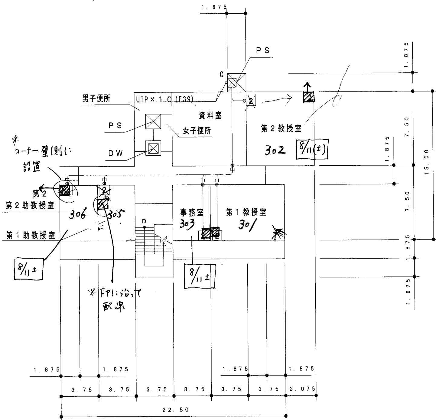
3 階 平 面 図
